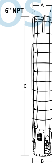
Acoplamiento NEMA 6"
