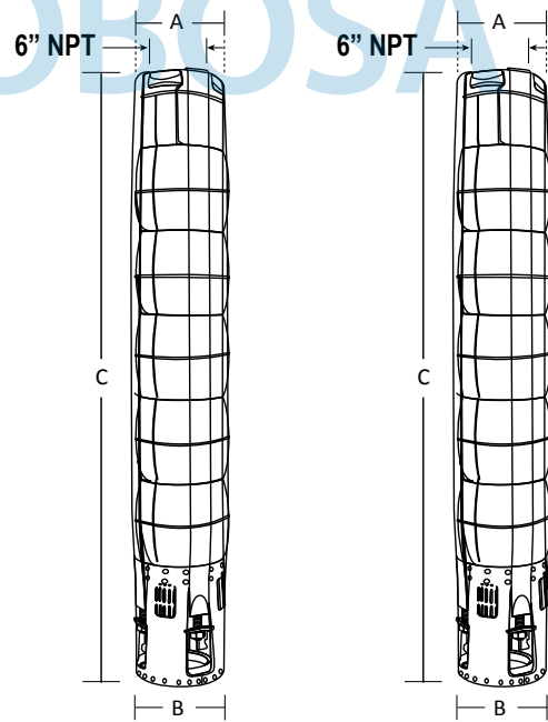
Acoplamiento NEMA 6" Fig. 1
