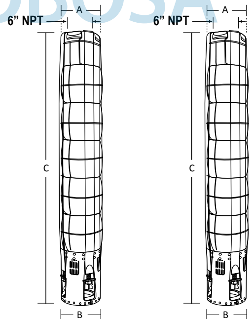
Acoplamiento NEMA 6" Fig. 1
