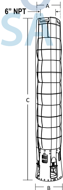
Acoplamiento NEMA 10" Fig. 2
