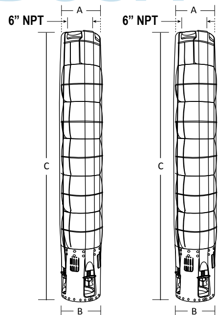
Acoplamiento NEMA 6" Fig. 1
