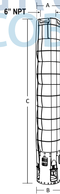
Acoplamiento NEMA 8" Fig. 1
