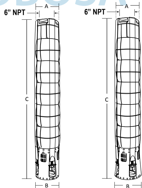
Acoplamiento NEMA 6" Fig. 1
