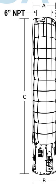
Acoplamiento NEMA 10" Fig. 2
