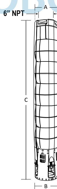
Acoplamiento NEMA 6" Fig. 1
